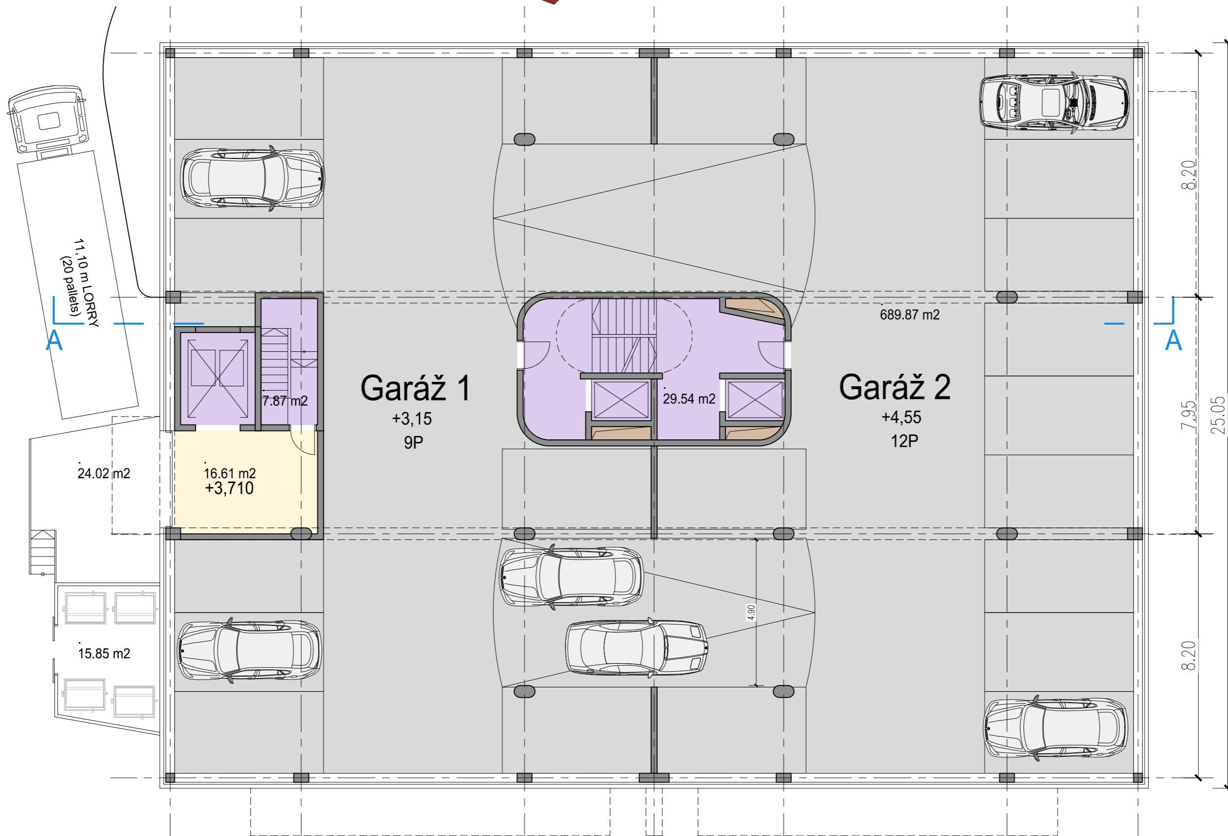
Pôdorys 2.NP
