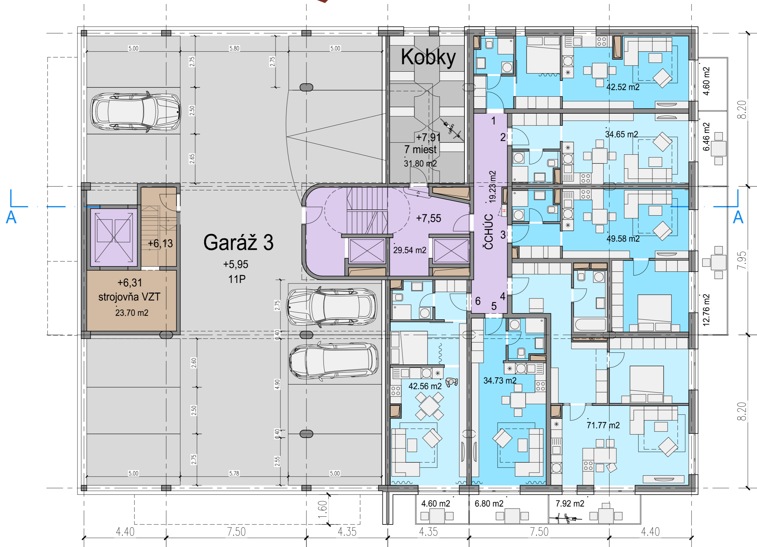
Pôdorys 3.NP
